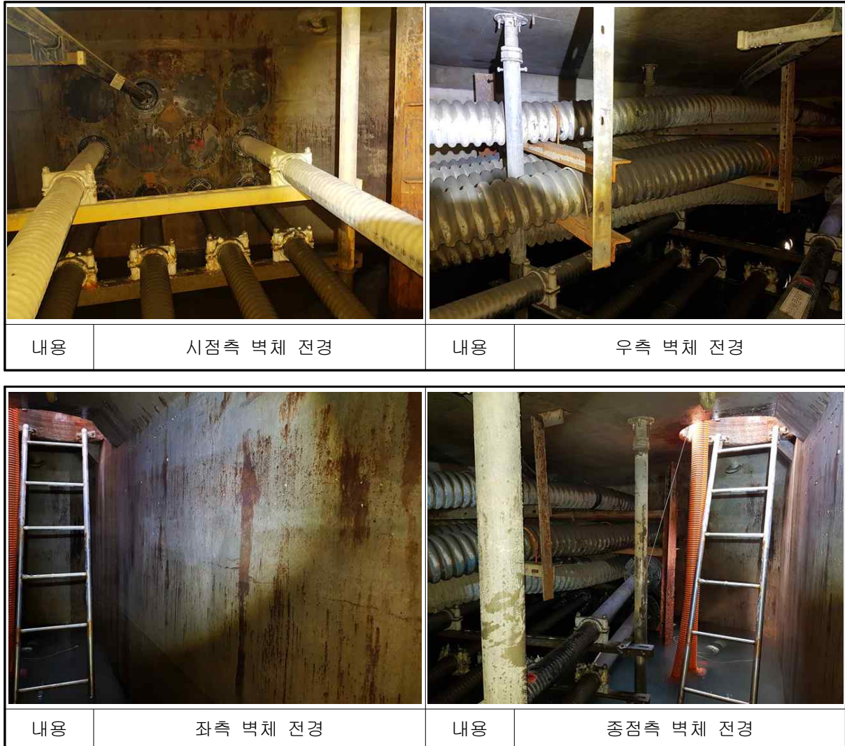
【사진 3.9】 운정~덕이 #0-1 전경
