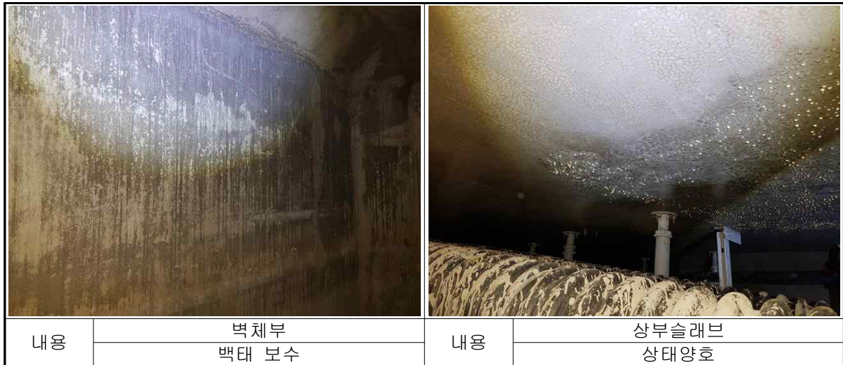
【사진 3.6】 맨홀 내부 주요 손상
